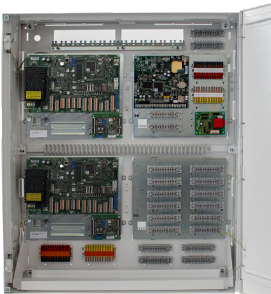
Gehäusotyp S110
