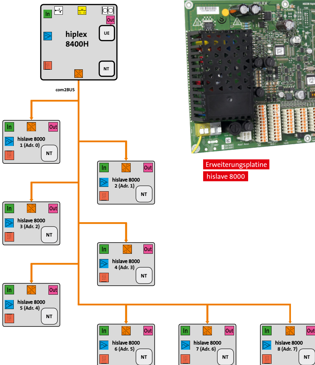
EMZ hiplex 8400H im Vollausbau mit 8 hislave 8000
