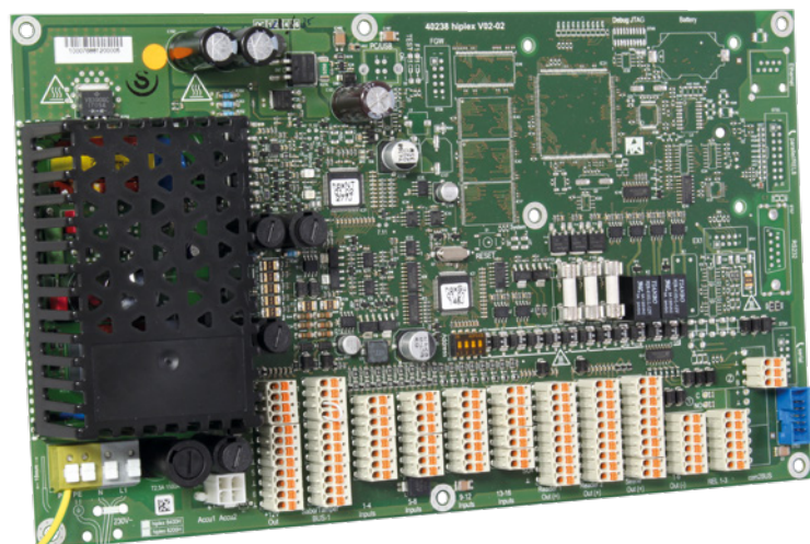
Erweiterungsplatine hislave 8000
